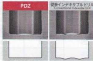
穴底形状イメージ Bottom Hole Shape Comparison φ20 被削材：S50C
