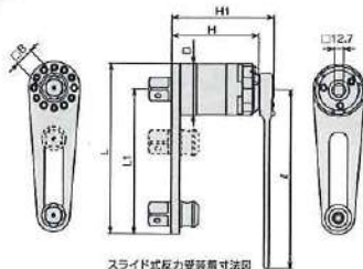
スライド式反力調整器寸法図
