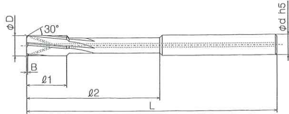
φ4.100 ~ φ20.100mm Y字オイルホール
